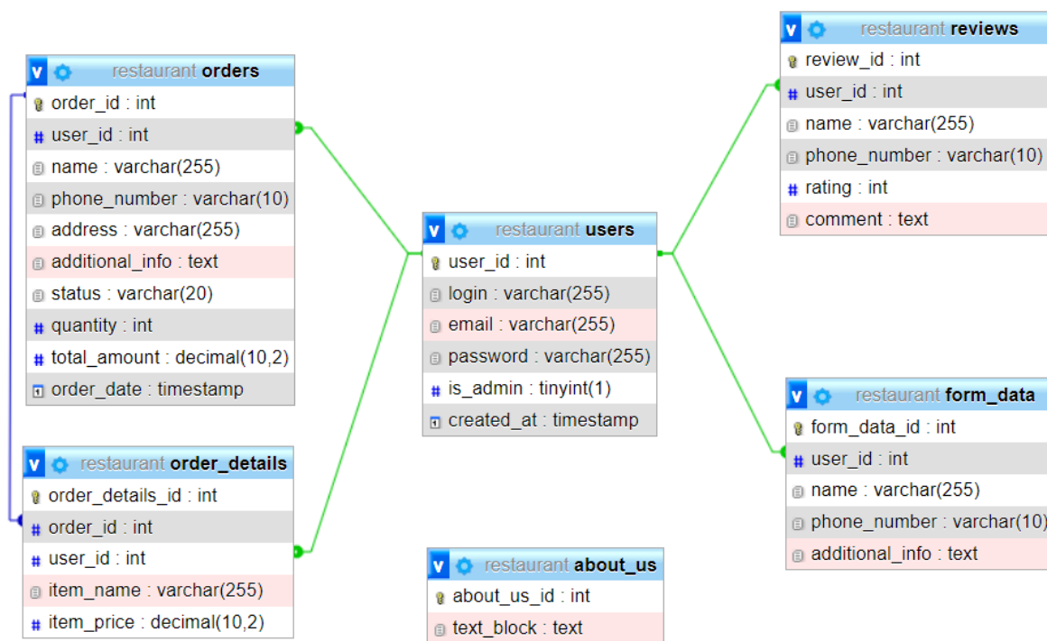
Рисунок 2.4 – Фізична модель бази даних web-додатку сервісу доставки замовлень з ресторану
