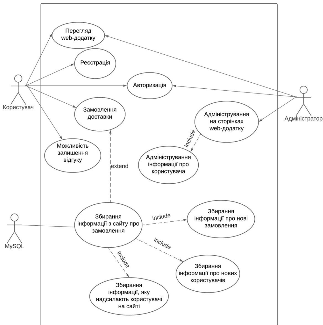
Рисунок 2.3 – Діаграма варіантів використання
