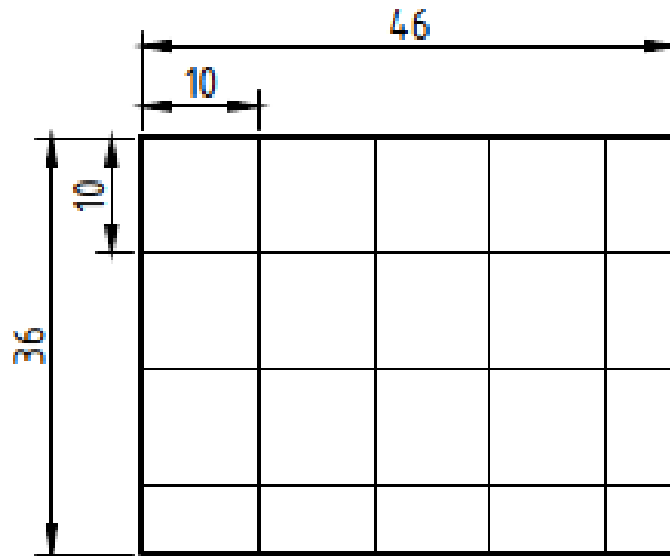
Рисунок 4.3 – Контур заземлення
