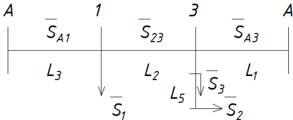
Рисунок 1.2 – Схема заміщення розрахункової схеми А
