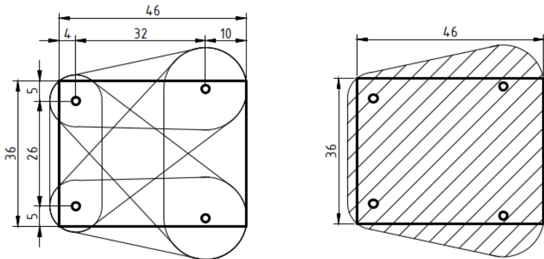
Рисунок 4.2 – Схема зони захисту від ураження блискавки підстанції на висоті h_x = 8 \text{ м}
