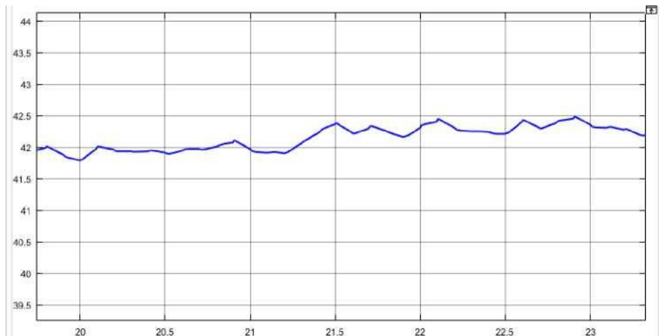
Рисунок 7.13 – Збільшений масштаб перехідної характеристики
