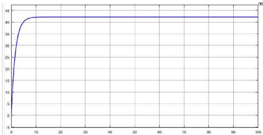
Рисунок 7.7 – Перехідна характеристика з ПД-регулятором
