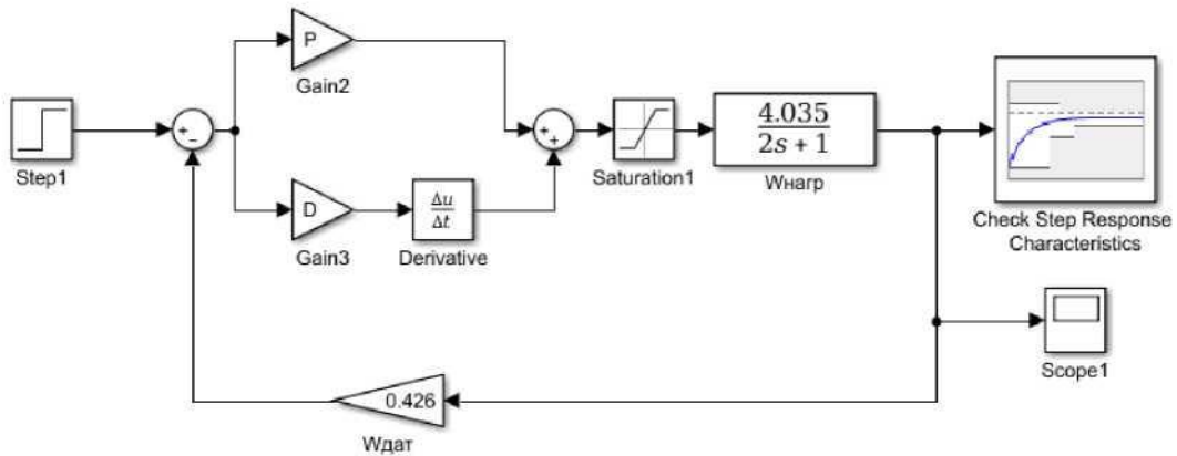
Рисунок 7.6 – Схема моделі з ПД-регулятором
