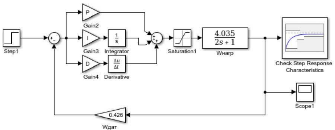
Рисунок 7.9 – Схема моделі з ПД-регулятором
