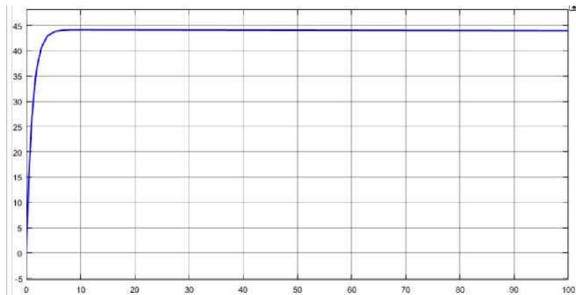
Рисунок 7.4 – перехідна характеристика з ПІ-регулятором
