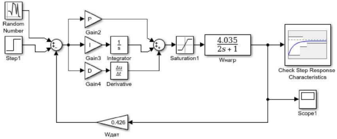
Рисунок 7.11 – Схема моделі зі збуренням
