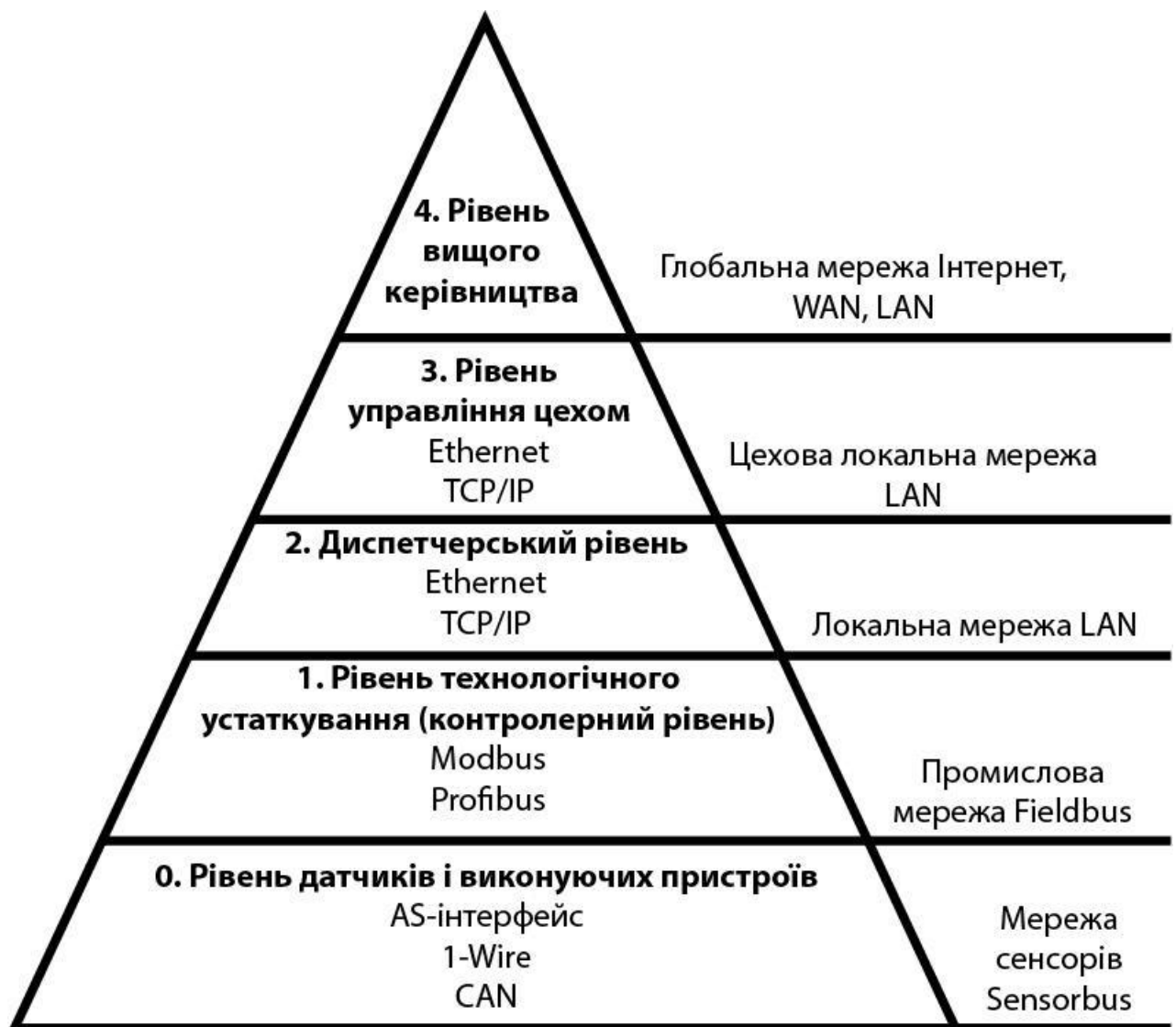
Рисунок 3.4 – Рівні ієрархії сучасної АСУ
