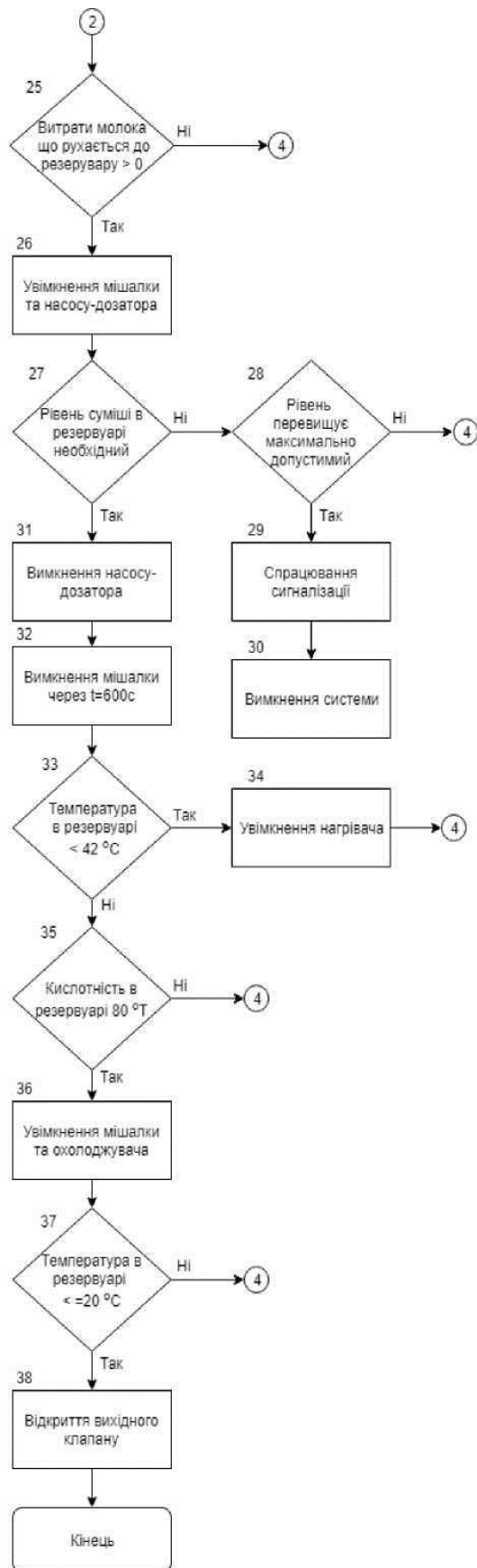
Рисунок 6.3 – Алгоритм процесу заквашування молока
