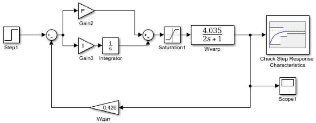
Рисунок 7.3 – Схема моделі з ПІ-регулятором
