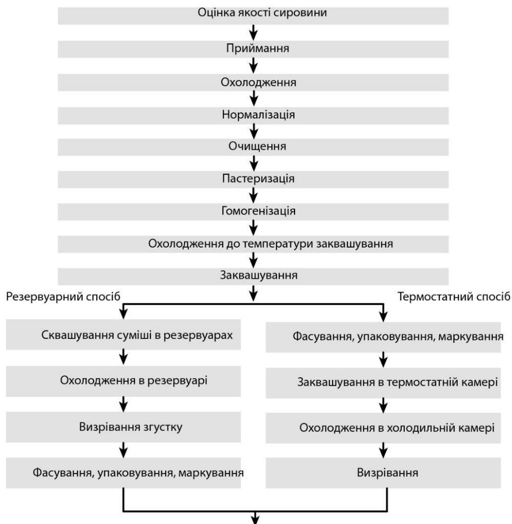
Рисунок 3.1 – Загальна схема технологічного процесу виготовлення йогурту
