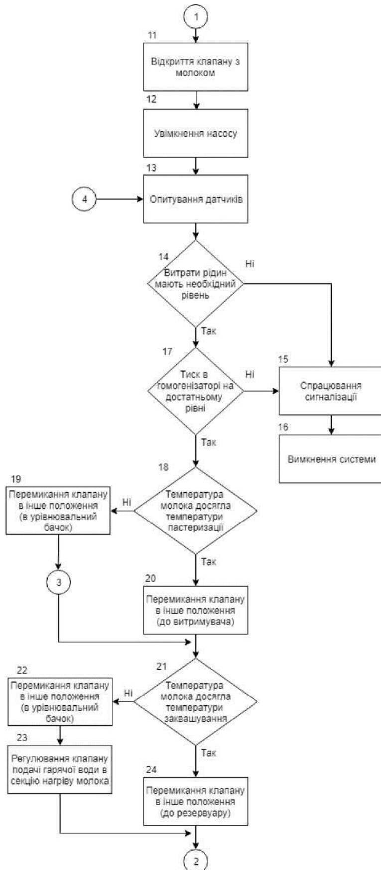
Рисунок 6.2 – Алгоритм управління процесом підготовки молока до заквашування
