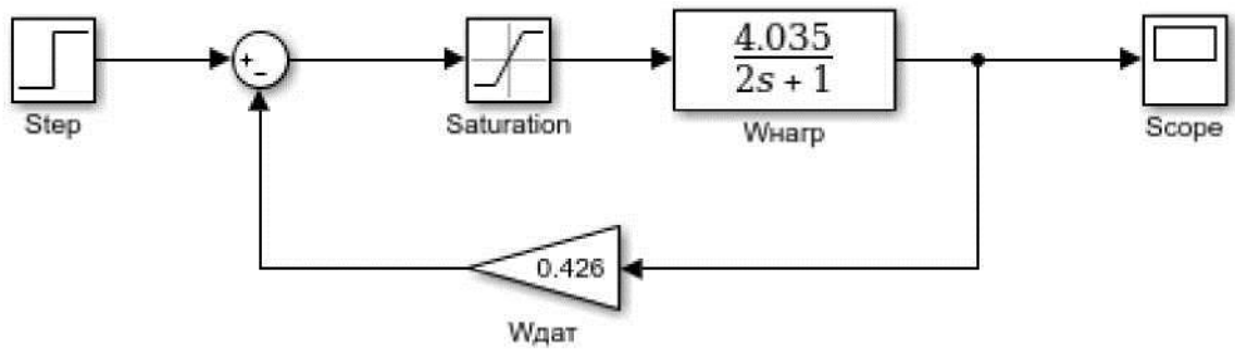
Рисунок 7.1 – Схема моделі
