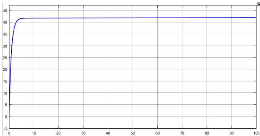
Рисунок 7.10 – Перехідна характеристика з ПД-регулятором
