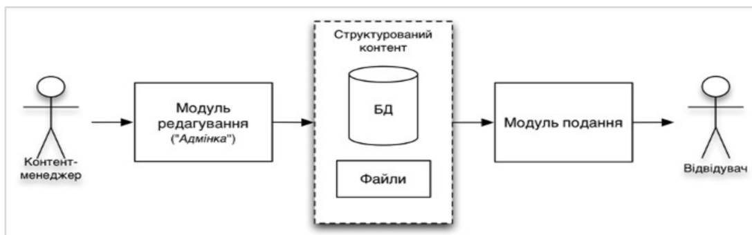
Рис. 2.2 – Структура CMS
