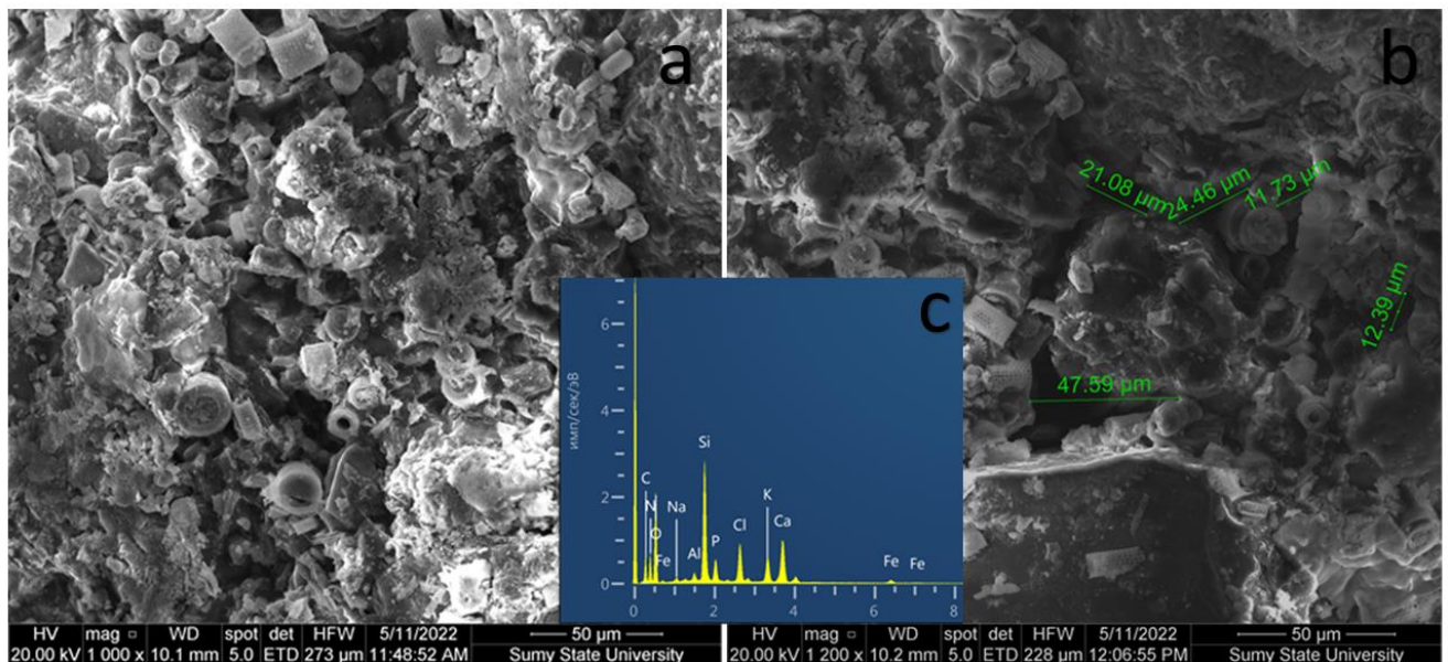
Рисунок 1.9 – SEM зображення морфології покриття карбамідної гранули: а) фосфатсвмісне покриття з додаванням діатоміту гранули карбаміду (збільшення \times 1000 ); б) розмір мікропор у покритті (збільшення \times 1200 ); в) EDX-спектр покриття
