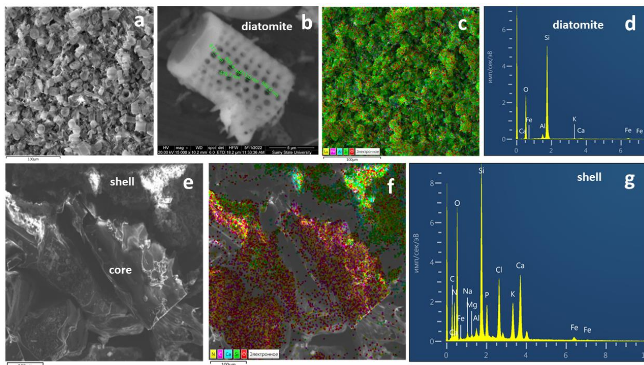
Рисунок 1.8 – SEM зображення морфології покриття карбамідної гранули: а) розмір частинок діатоміту (збільшення \times 1000 ), б) розмір пор деяких частинок діатоміту (збільшення \times 15000 ), в) розподіл елементів в діатоміті; д) спектр EDX діатоміту; е) фосфатвмісне покриття з додаванням діатоміту гранули карбаміду (збільшення \times 1000 ); ф) розподіл елементів в оболонці гранул; г) EDX-спектр покриття
