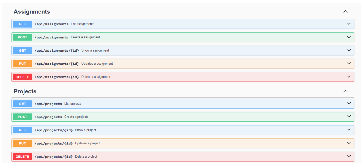
Рисунок 3.5 – UI документація маршрутів Assignments та Projects
