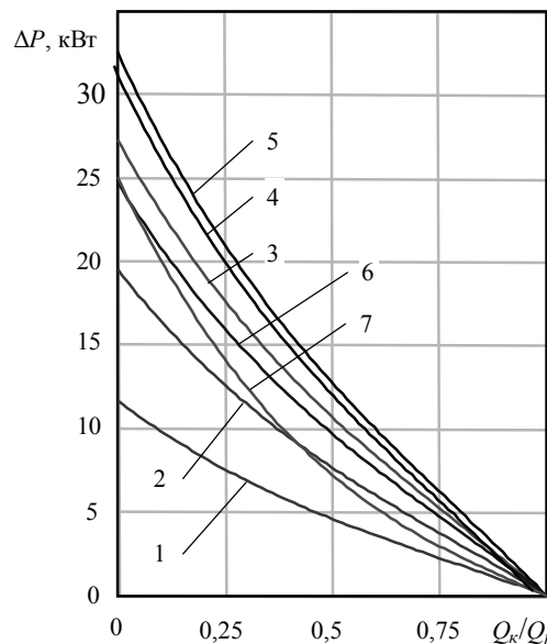
Рис. 2. Залежність плати за реактивну потужність від ступеня КРП
