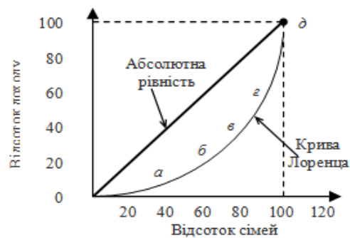
Рис. 1 Крива Лоренца
