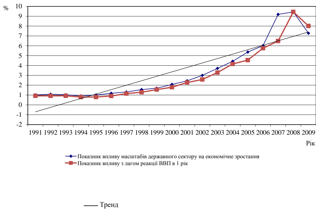
Рис. 3. Вплив масштабів державного сектору на економічне зростання в Україні за період 1991-2009 рр., власні розрахунки
