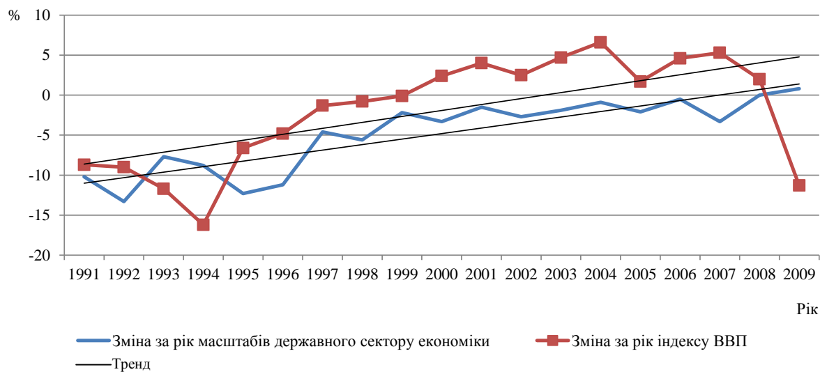
Рис. 2. Зіставлення показників абсолютного приросту індексу ВВП та інтегрального коефіцієнту масштабу державного сектору економіки України за 1991-2009 рр., власні розрахунки
