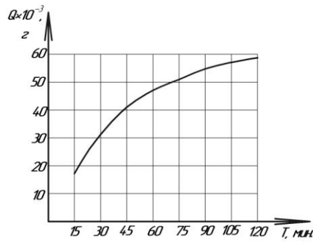
Малюнок 3 – Залежність знімання металу від тривалості обробки
