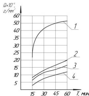
Малюнок 2 – Вплив типу абразивного середовища на знімання металу: 1- шліфзерно; 2 - формокорунд - циліндр; 3 - ПТ-10; 4 - волзький пісок
