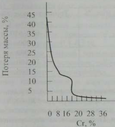
Рисунок 27 – Относительная скорость окисления сплавов на воздухе (48 часов, 1000^{\circ}\text{C} ) в зависимости от содержания хрома в сплаве
