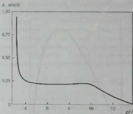
Рисунок 20 – Влияние pH на скорость коррозии железа в воде
