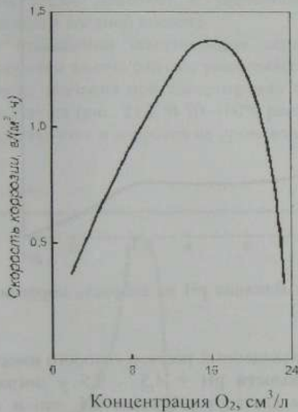
Рисунок 19 — Влияние концентрации кислорода на скорость коррозии стали в дистиллированной воде при 25 0 С
