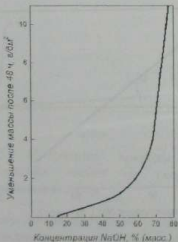
Рисунок 23 — Зависимость скорости коррозии листового железа в кипящих растворах NaOH от их концентрации
