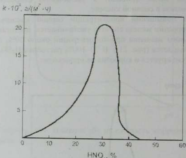
Рисунок 22 – Влияние концентрации \text{HNO}_3 на скорость малоуглеродистой стали
