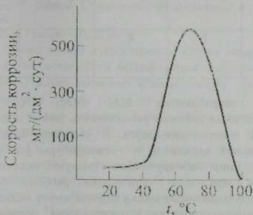
Рисунок 33 – Влияние температуры на скорость коррозии Zn в дистиллированной воде
