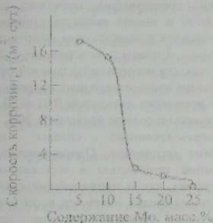
Рисунок 31 – Зависимость скорости коррозии сплава Ni–Mo в 10% HCl при 70 0 C от содержания молибдена
