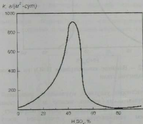
Рисунок 21 – Влияние концентрации H_2SO_4 на скорость коррозии железа
