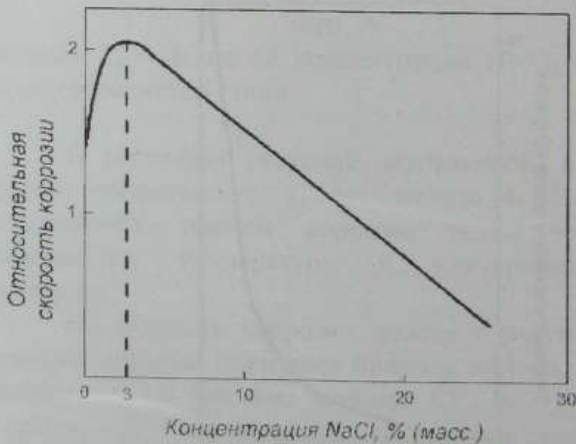
Рисунок 24 – Влияние концентрации нейтрального раствора соли (NaCl) на скорость коррозии железа при 18 0 С
