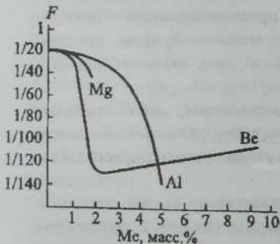
Рисунок 29 – Влияние добавок магния, бериллия и алюминия на скорость окисления меди на воздухе при 800^{\circ}\text{C} .
