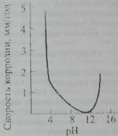
Рисунок 32 – Влияние pH на коррозию Zn
