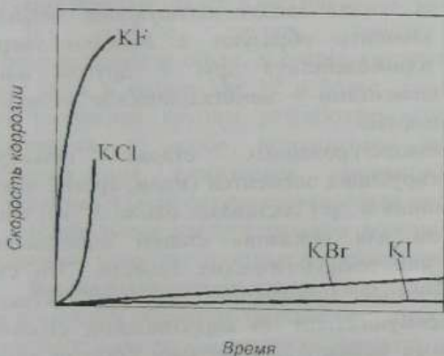
Рисунок 25 — Влияние природы аниона солей галогеноводородных кислот на скорость коррозии железоуглеродистых сплавов
