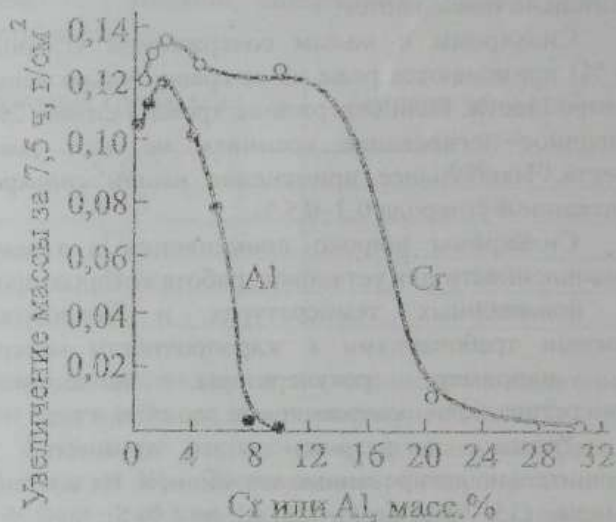
Рисунок 28 – Зависимость скорости окисления сплавов Fe–Cr и Fe–Al на воздухе при 1200 0 C от содержания в сплаве легирующего компонента
