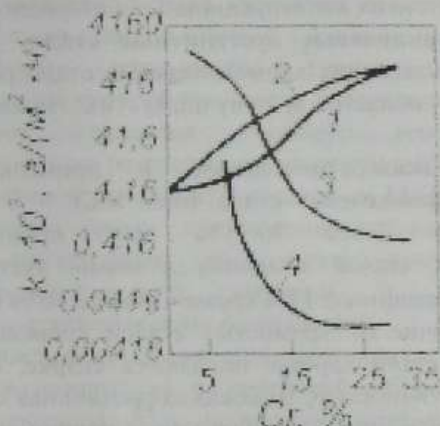
Рисунок 26 – Влияние содержания хрома на скорость коррозии стали в растворах кислот:
