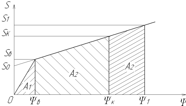
Рисунок – Диаграмма истинных напряжений: S_0 – экстраполированный предел текучести; S_\theta – истинное напряжение в момент образования шейки; S_k – истинное сопротивление разрушению; \psi_\theta и \psi_\kappa – относительное сужение в момент образования шейки и разрушения.
