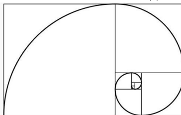
Рис. 2 Спіраль Фібоначчі
