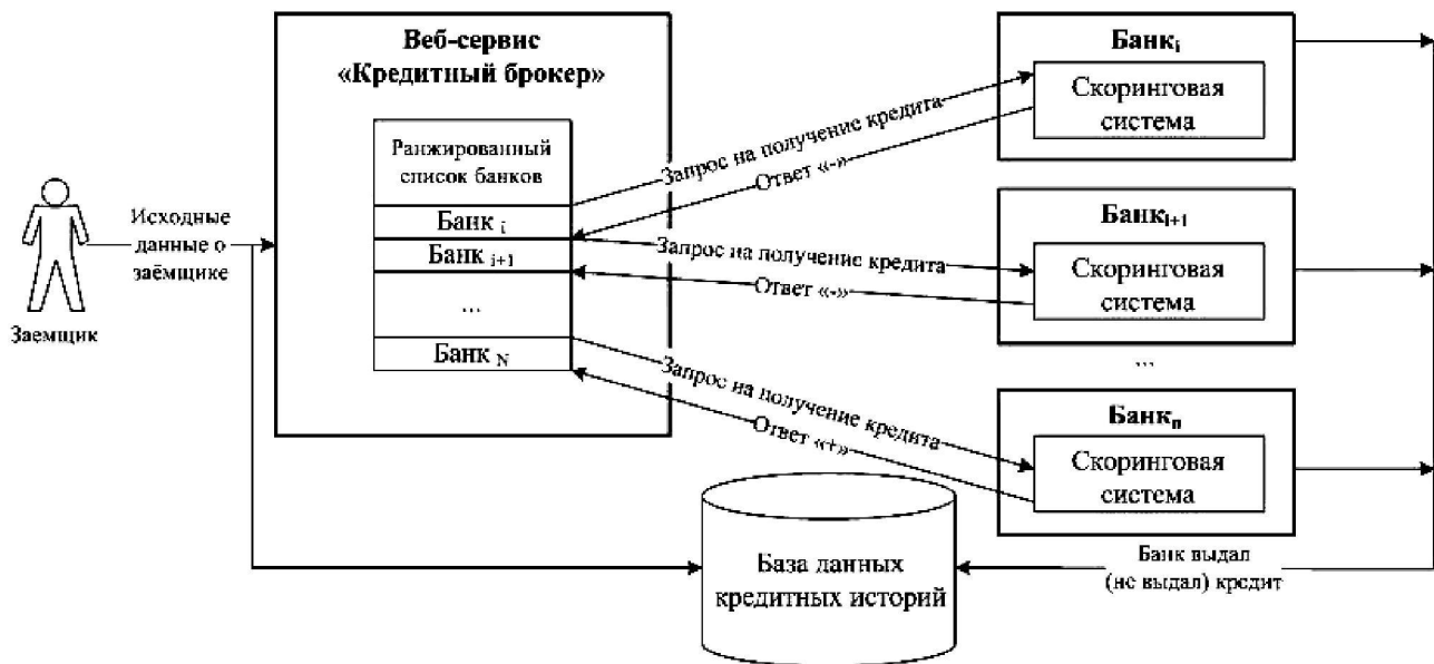
Рис. 5. Интеграция веб-сервиса "Кредитный брокер" со скоринговыми системами и базой данных кредитных историй
