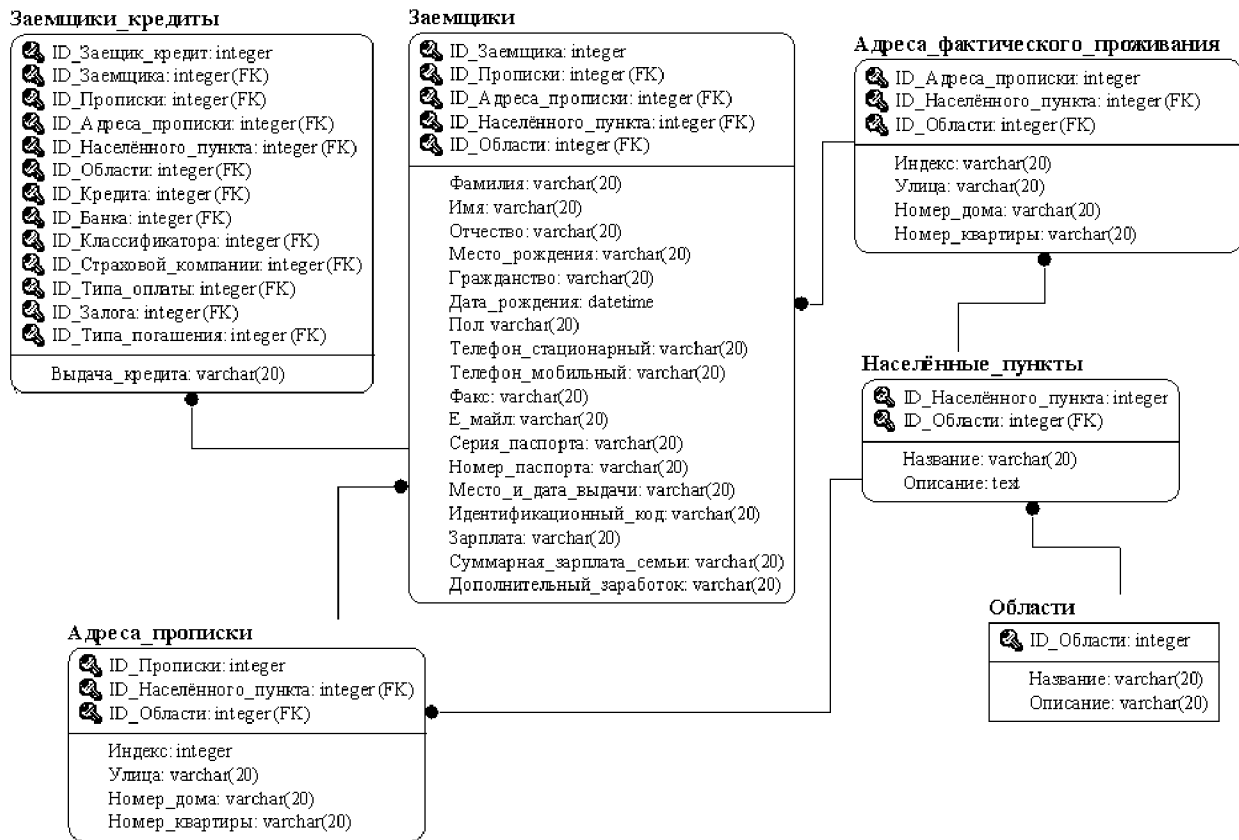
Рис. 3. Структура базы данных кредитной статистики
