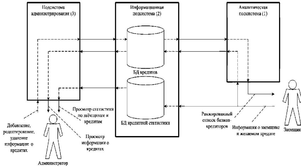
Рис. 1. Архитектура веб-сервиса “Кредитный брокер”
