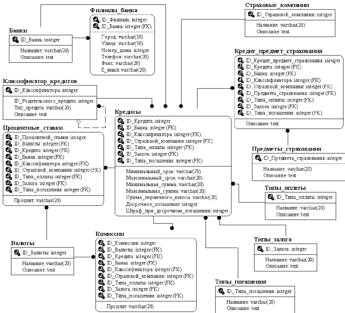
Рис. 2. Структура базы данных кредитов для физических лиц
