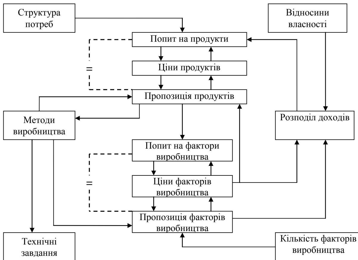
Рис. 2 – Схема моделей загальної рівноваги
