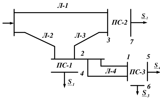
Початкова схема мережі
