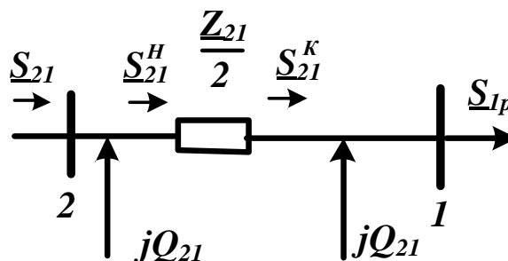
Рисунок 1.8 Схема заміщення лінії Л-4
