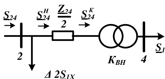
Рисунок 1.5 – Схема заміщення підстанції ПС – 1
