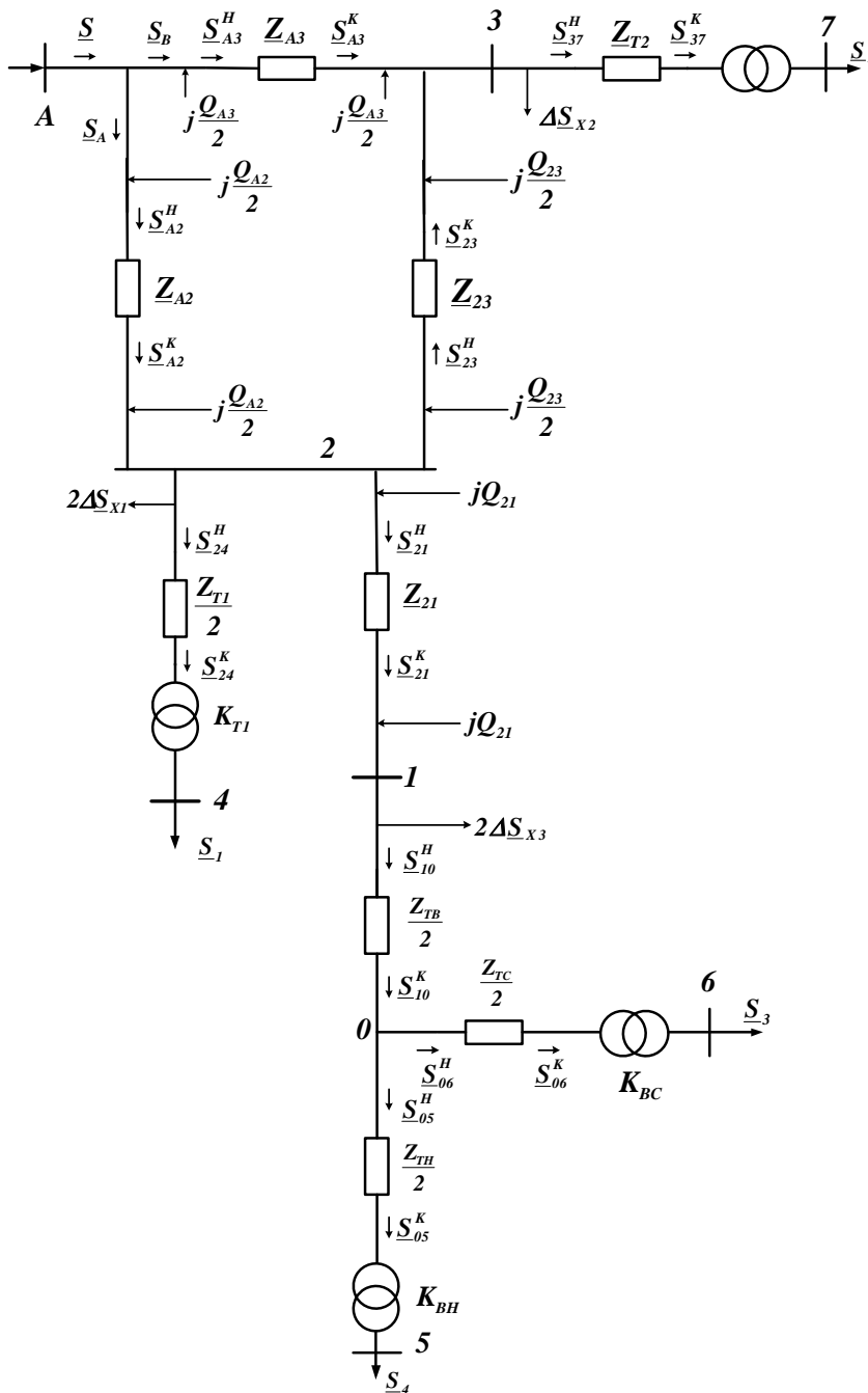
Схема заміщення мережі
