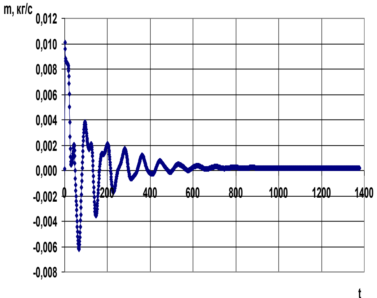
Рисунок 2.3 Збіжність результатів
