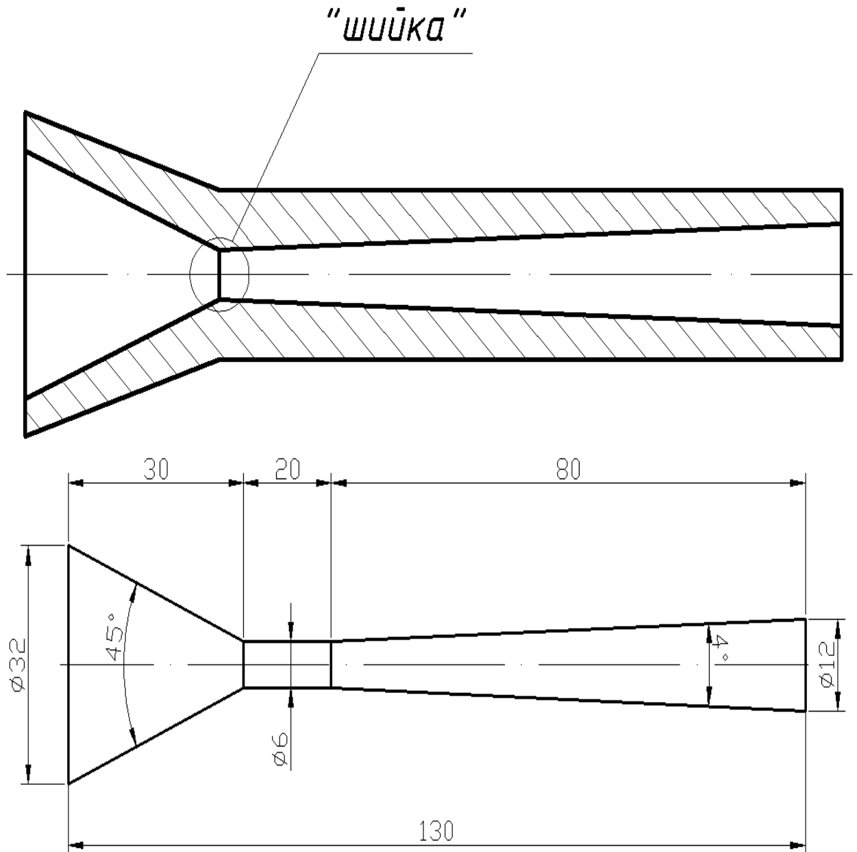
Рисунок 3.10 Переріз сопла форми Вентурі абразивоструменевої машини
