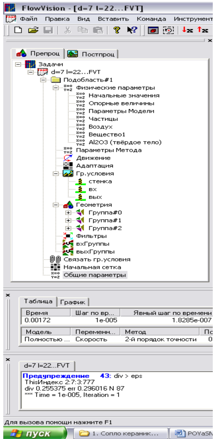
Рисунок 2.7 Дерево препроцессора
