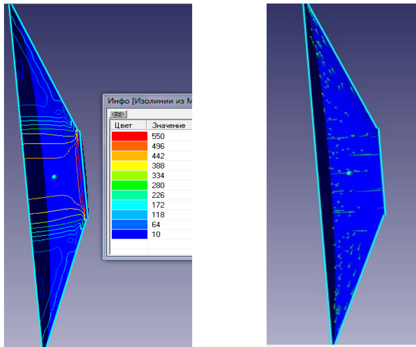
Рисунок 3.8 Візуалізації течії конічного сопла
